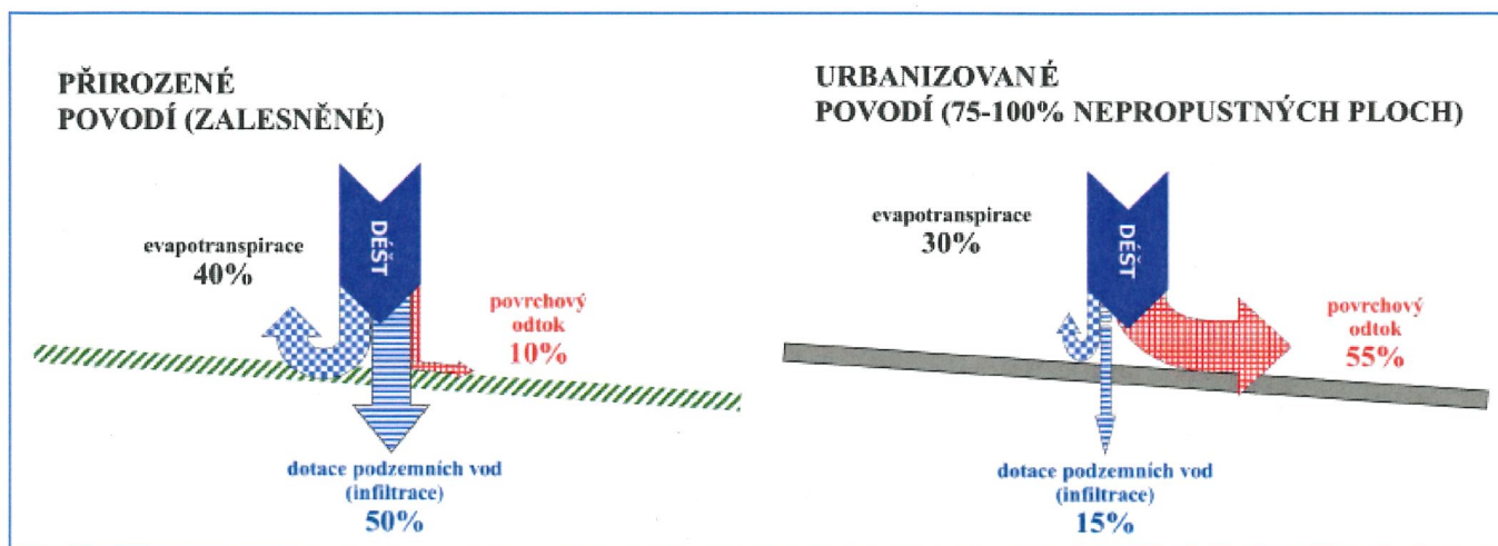
Obrázek 1 Porovnání zvýšení odtoku z povodí přirozeného a urbanizovaného (Stránský, 2013)
