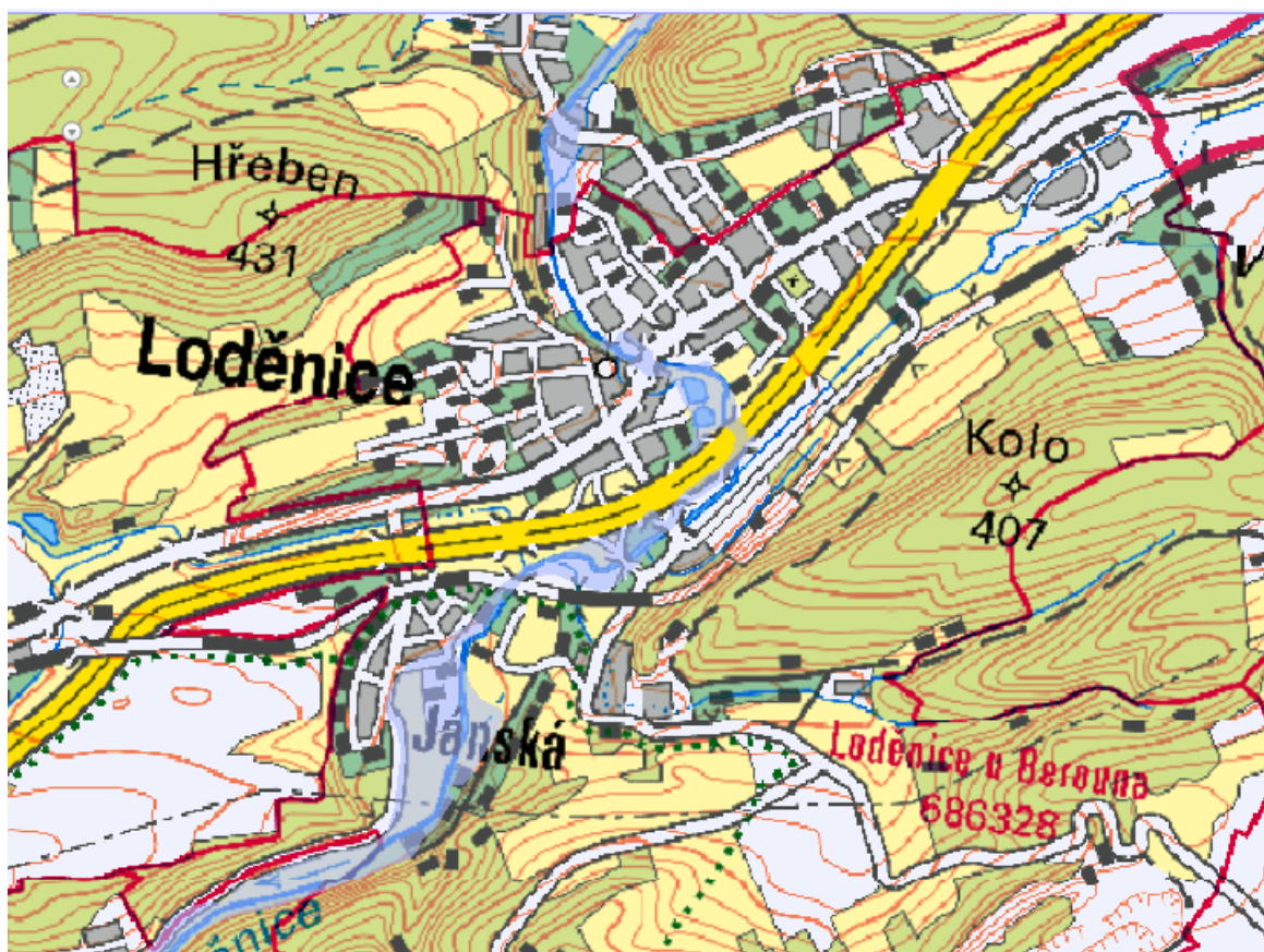
Obrázek 3: Záplavové území obce
